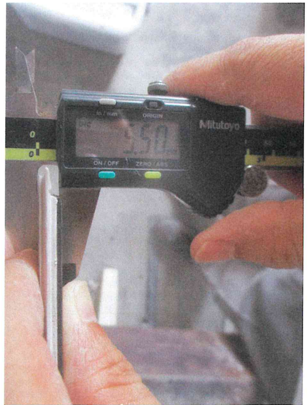
照片 2 試驗件各組件尺寸查核
